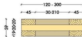
Schnitt B
